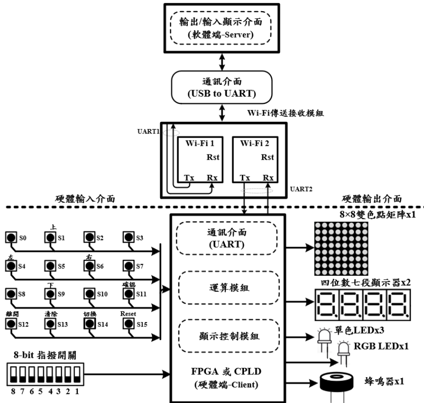
圖 1、系統架構圖
